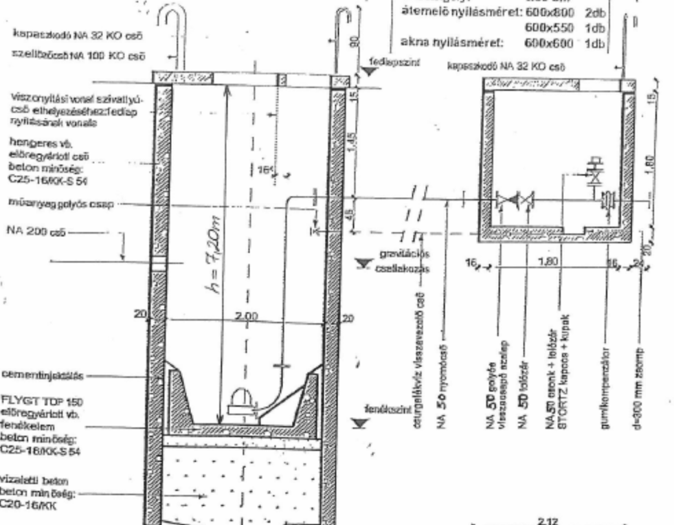
METSZET M 1:50
